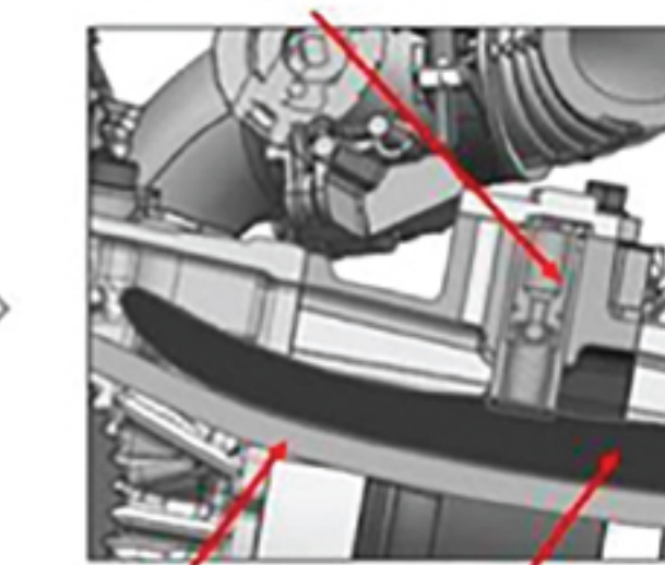
Xích cam Thanh dẫn hướng xích cam
